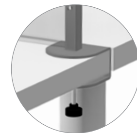
Schraubklemmbefestigung für Tischplatten bis zu 4,7 cm.
